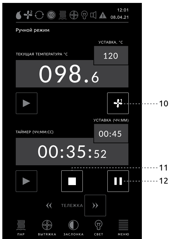
Рисунок 18 - Пример экрана ручной выпечки в процессе работы
