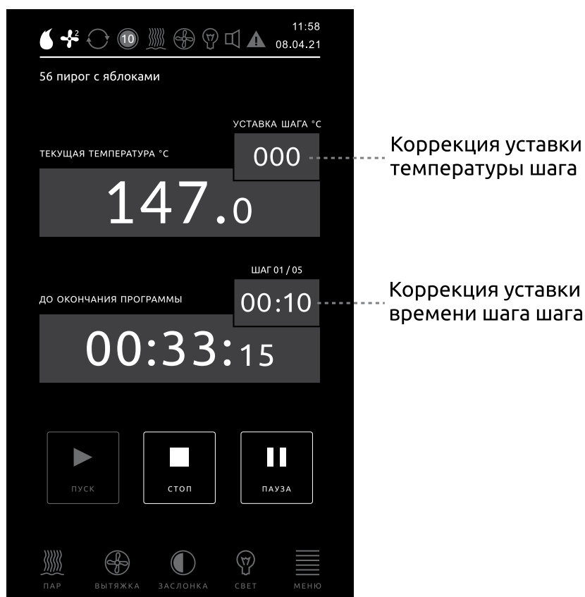
Рисунок 5 - Коррекция уставок температуры и времени
