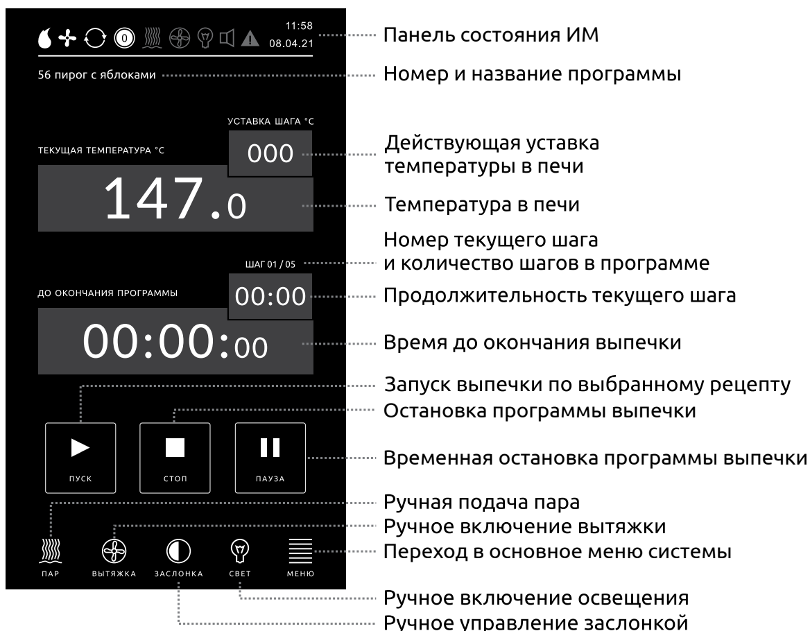
Рисунок 2 - Главный рабочий экран автоматического режима работы
